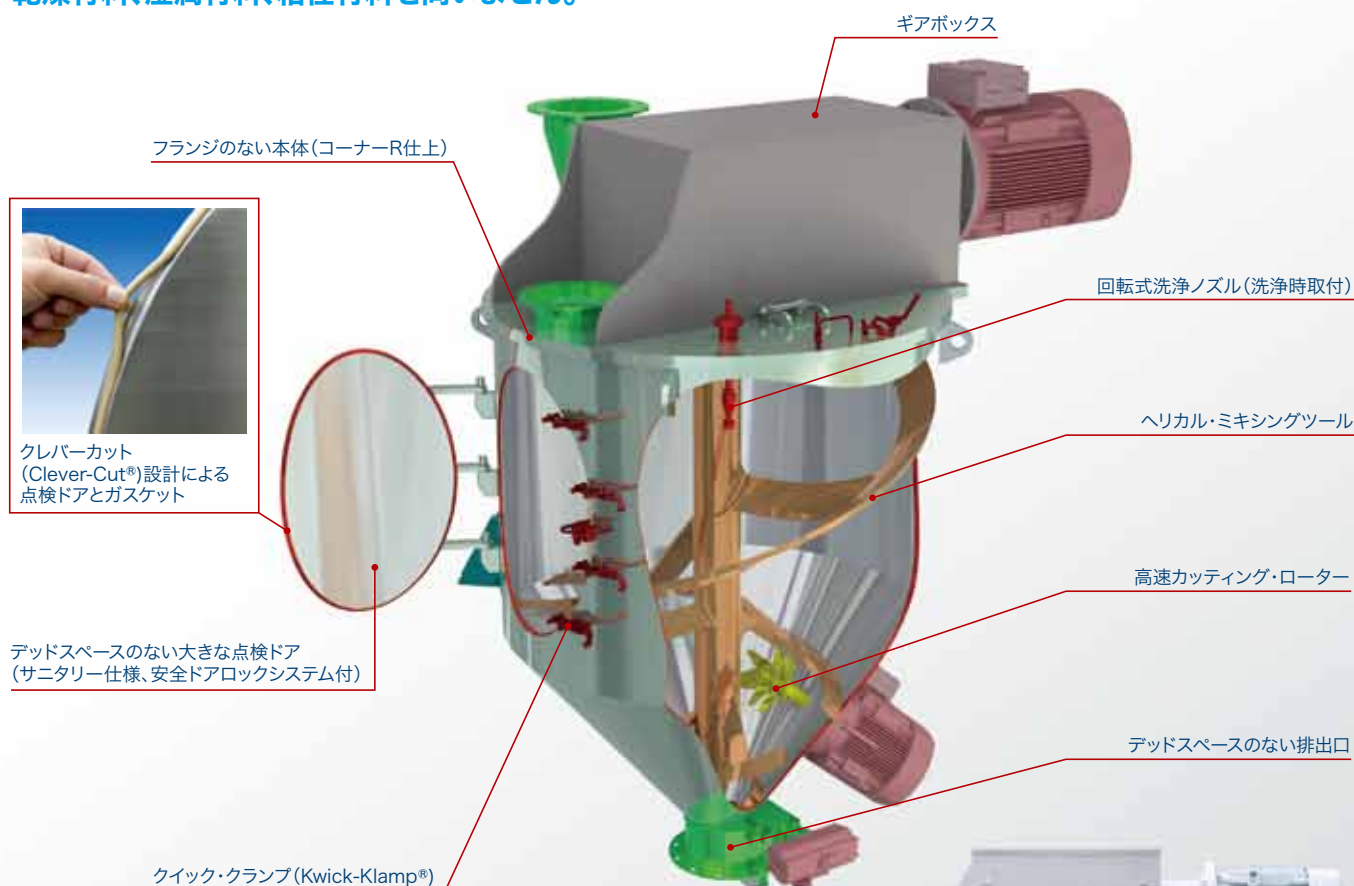
ヘリカル・ミキシングツール
