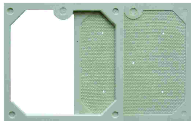
板框式滤板 Plate & frame type
