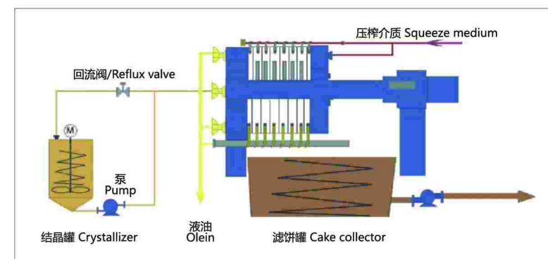
过滤和压榨过程 Filtration & squeeze process
