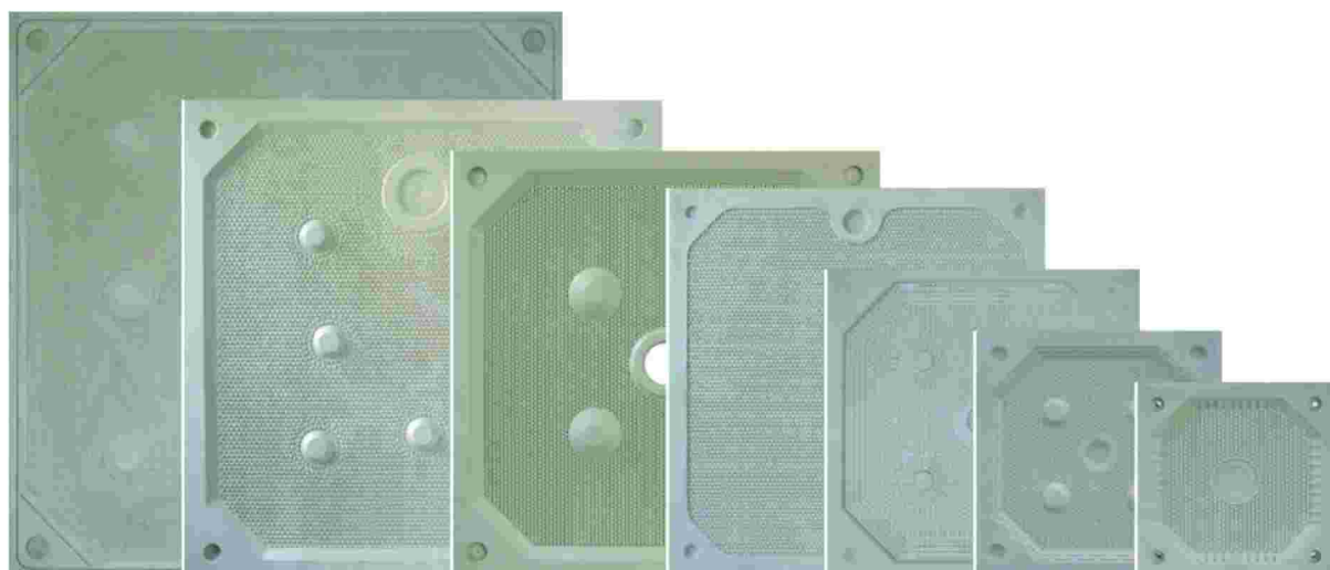
▲ 400mm系列—2000mm系列厢式滤板 Recessed chamber plates range 400mm to 2000mm series
