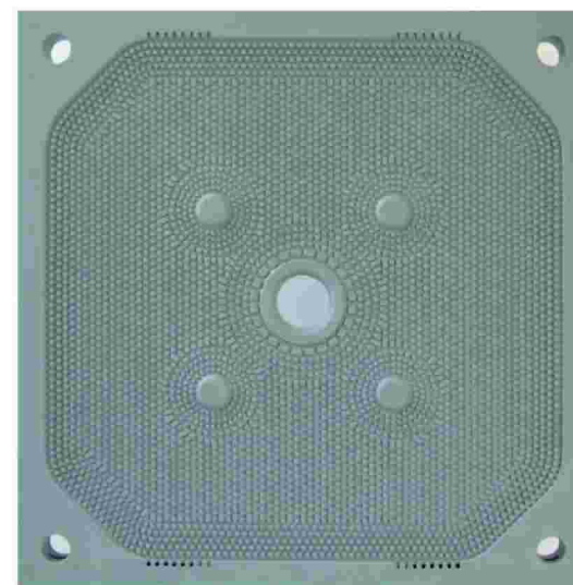
聚丙烯隔膜滤板 PP membrane plates
