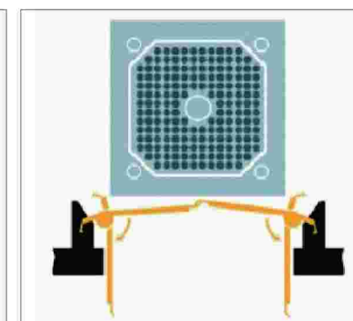
集液翻板 Drip tray
